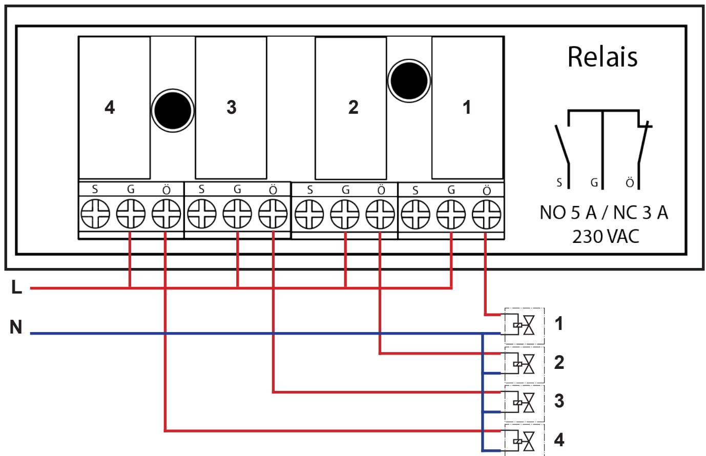
Bovenstaande toepassing met 4 kleppen NO
