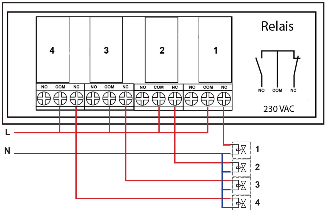
Bovenstaande toepassing met 2 tot 4 floatswitches. (max. 4x enkel of 2x dubbel)
