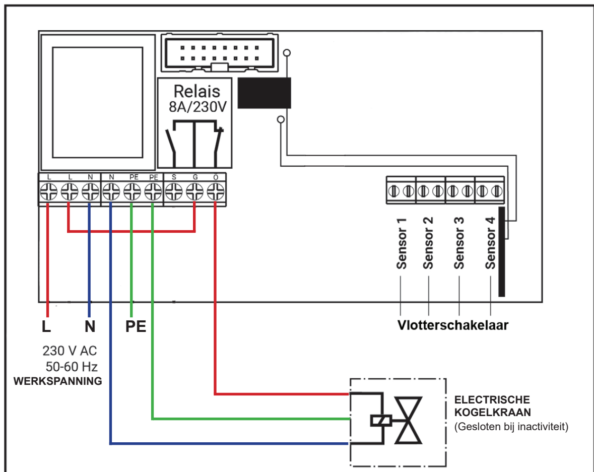
Bovenstaande toepassing met 1 floatswitch (max. 1x enkel)
